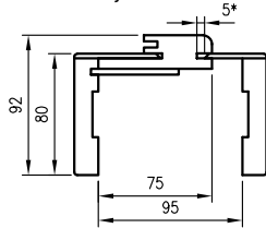
Przekrój poziomy ORB
