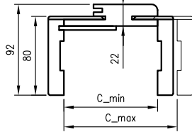
Przekrój ORB 075
