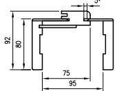
Przekrój ORB 075
