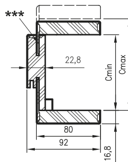
Przekrój stojaka
